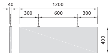
Módulo 1200 x 400mm
