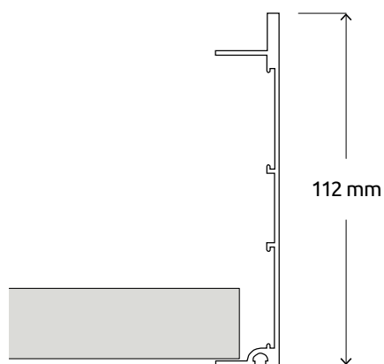
Perfil Gridline Aluminio Integra/Tegular 24 55 14 11 H
